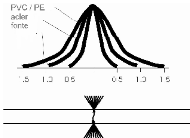
Figure 13 : Diffusion du bruit en fonction du matériau
