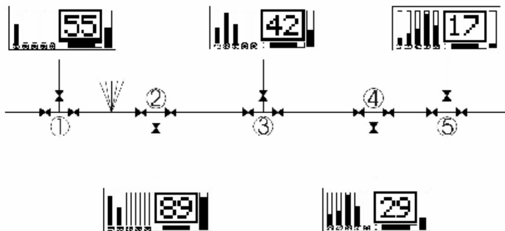
Figure 12 : Localisation d'une fuite
