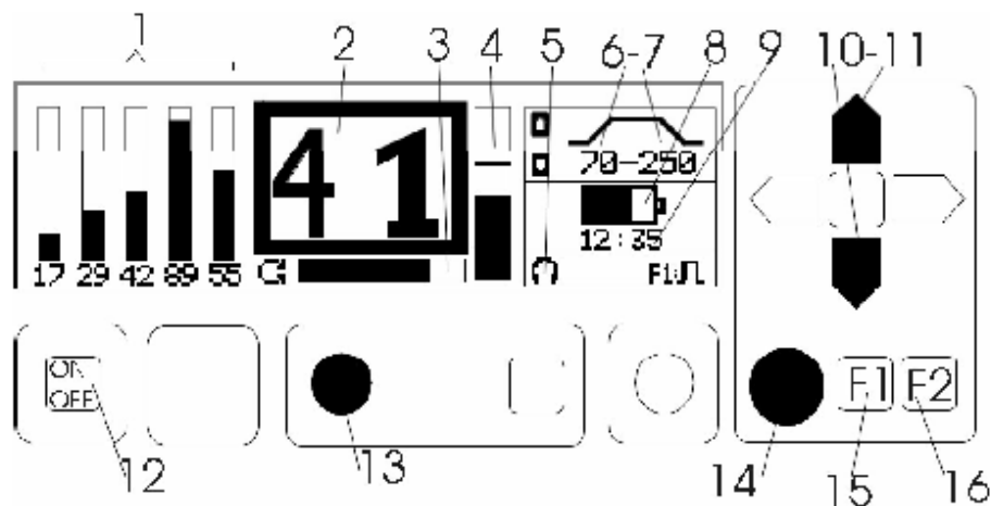
Figure 11 : Représentation - Mesure au géophone
