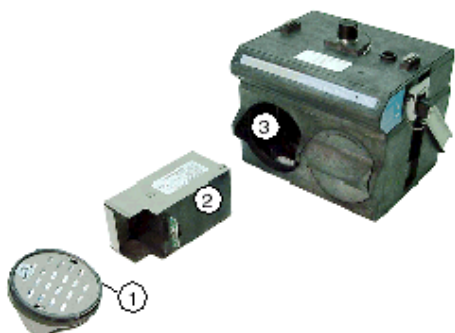
Figure 1-4 Composants de batterie du bloc 2191EX
