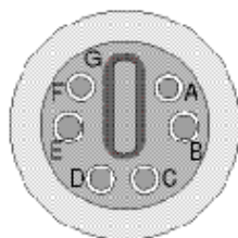
Figure 1-7 2150EX – Broches du connecteur de communication
