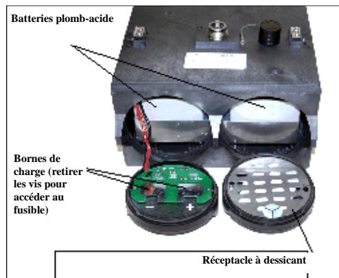
Figure 4-2 Bornes de charge du bloc 2196EX
