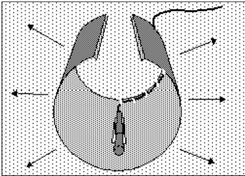
Figure 2-7 Sonde de débit installée sur un collier élastique
