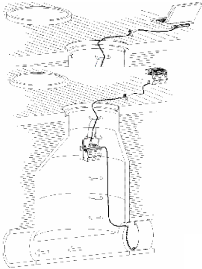
Figure 2-1 Installation classique dans une canalisation circulaire raccordée à un ordinateur portable
