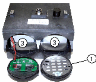
Figure 1-5 Composants de batterie du bloc 2196EX
