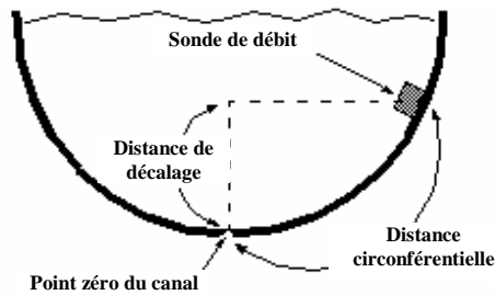
Figure 3-3 Mesure du décalage par rapport au niveau zéro
