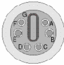
Figure 1-7 2150EX – Broches du connecteur de communication
