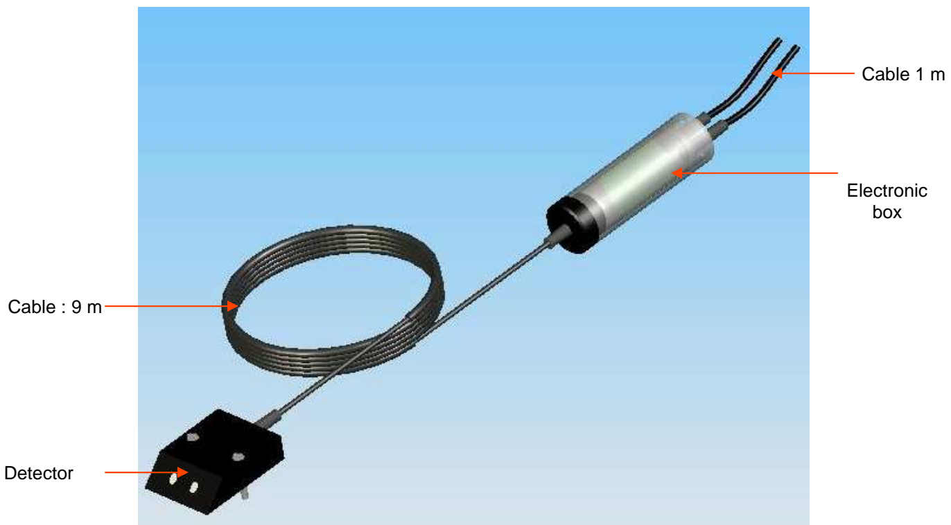
level actuator
